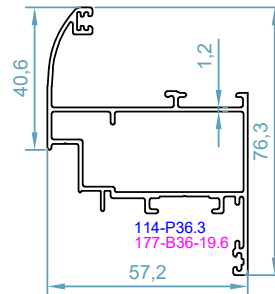
code : 1543 پنجره داخل بازشو Inward Opening Window weight : 1.01 kg/m
