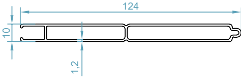
code : 2520 ورق تک جداره Shutter Profile weight : 0.82 kg/m
