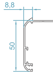
code :2500 پروفیل روکوب border profile weight 0.39 kg/m
