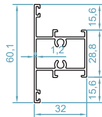
code : 1620 سپری لنگه زهوار دار T profile for sash weight : 0.71 kg/m
