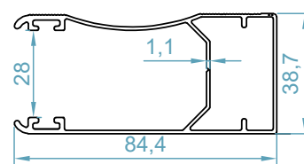
ریل الگانس Elegance Rail Profile code: 9152
