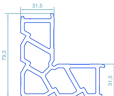
code : 113 گونیای پانچی Corner Cleat weight : 4.13kg/m
