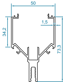
code : 3151 آداپتور کنج بیرونی 90° Corner Adapter Profile 90° weight : 1.23kg/m
