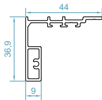
code : 2119 آداپتور سه لنگه وسط باز شو قفل شو Adapter Profile weight : 0.55 kg/m
