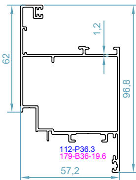
code : 1540 درب داخل بازشو Inward Opening Door Sash weight : 1.19 kg/m
