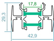
code : 2321-2321 وسط چهار لنگه Adjoining Sliding Sash Pr. weight : 0.9 kg/m
