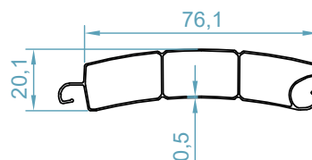
تیغه دوپل جدید New Dopol Shutter
