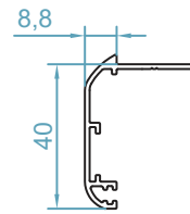
code :2501 پروفیل روکوب border profile weight 0.36 kg/m
