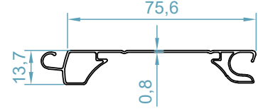
تیغه تک جداره رو به بیرون Single Sheet Shutter code: 9002
