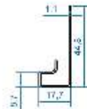
code : 3149 بروزگیر مسیله نو عمودی Dilatation Isolation Prof weight : 0.284 kg/m
