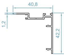
code : 2118 پروفیل اینترلاک Interlock Profile weight : 0.4 kg/m
