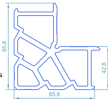
code : 179 PC B42 قابل تولید در اندازه های مختلف
