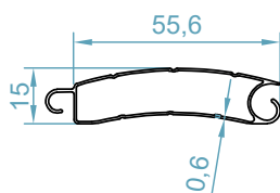
تیغه قوس 60 60 Curve Shutter
