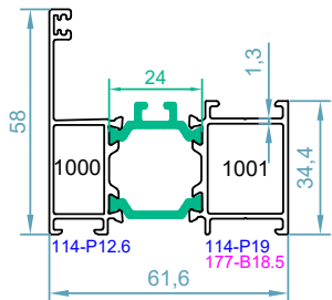
code : 1000-1001 پروفیل فریم Frame Profile weight : 1.22 kg/m
