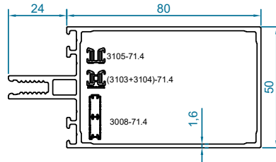
code : 3057 پروفیل افقی Transom Profile weight :1.67kg/m J_x=19.2 \text{ cm}^4 J_y=65.5 \text{ cm}^4
