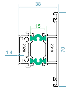
code : 2319-2320 سپری زهواردار T profile weight :1.00 kg/m J_x=8.77 \text{ cm}^4 J_y=6.19 \text{ cm}^4
