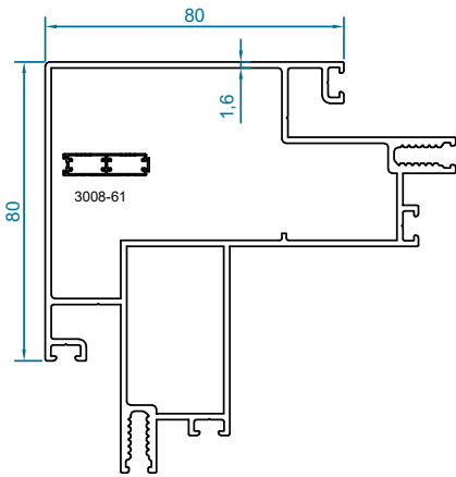
code : 3143 پروفیل کنج بیرونی 90° Corner Profile 90° weight : 2.7kg/m J_x = 101.16 \text{ cm}^4 J_y = 98.93 \text{ cm}^4
