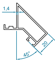
code : 3139 آداپتور کنج داخلی 90° Corner Adapter Profile 90° weight : 0.62kg/m
