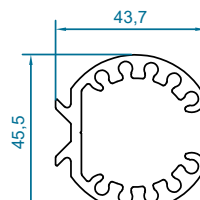
code : 3106 كانكتور زاویه در افقی Angular Joint Profile weight :0.36kg/m
