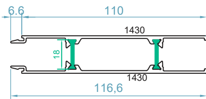
code :1430-1430 ورق دو جداره ی ترمال بریک Thermal break facade weight : 1.5 kg/m
