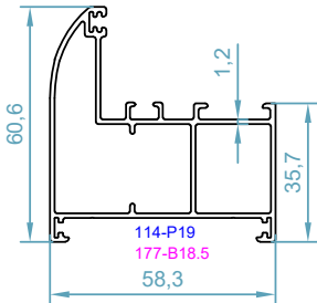
code : 1501 پروفیل فریم Frame Profile weight : 1.02 kg/m
