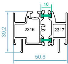
code : 2316-2317 آداپتور وسط چهار لنگه sash inversion profile weight :1.25 kg/m Jx=10.1 \text{ cm}^4 Jy=5 \text{ cm}^4
