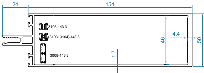
code : 3062 پروفیل افقی Transom Profile هم راستا با عمودی 3002 weight :2.71kg/m J_x=34.2 \text{ cm}^4 J_y=357.2 \text{ cm}^4
