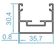
code : 2549 فریم توری پلیسه fly screen frame weight :0.430 kg/m
