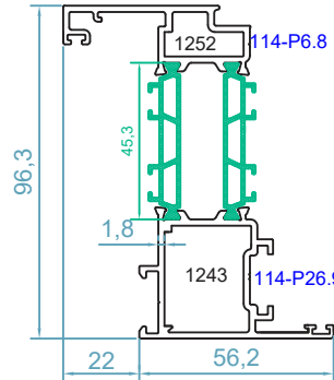
code : 1243-1252 لنگه پنجره sash profile weight 2.09 kg/m
