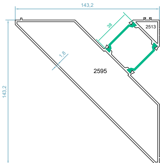
code :2513-2595 آداپتور کنج فیکس مونو ریل Corner Adapter weight 3.18kg/m
