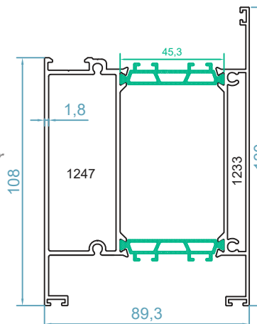
code : 1020-1256 اداپتور درب بیرون بازشو outward opening adapter weight 1.68 kg/m
