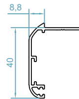
code :2501 پروفیل روکوب Border Profile weight : 0.35 kg/m
