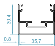
code : 2549 فریم توری پلایسه fly screen frame weight : 0.43 kg/m
