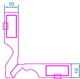
code : 176 PC B10 گونیا آلنی فریم طول برش 26 میلی متر
