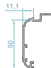
code :2558 پروفیل روکوب border profile weight 0.39 kg/m
