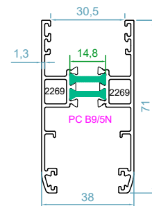
code : 2269-2269 لنگه بدون زهوار Sash Profile weight :1.14 kg/m J_x=9.4 \text{ cm}^4 J_y=15.4 \text{ cm}^4
