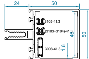
code : 3059 پروفیل افقی Transom Profile weight :1.39kg/m J_x=13.6 \text{ cm}^4 J_y=25.15 \text{ cm}^4
