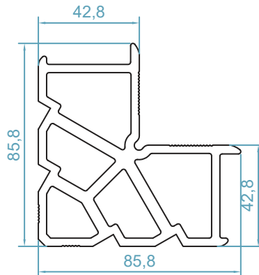
code : 112 گونیا پانچی corner cleat weight 5.00kg/m
