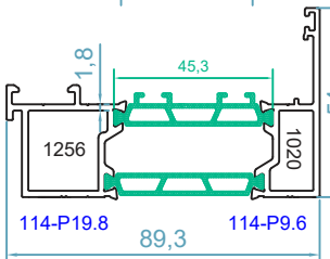
code : 1020-1256 اداپتور درب بیرون بازشو outward opening adapter weight 1.68 kg/m
