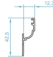
code : 2508 ریل توری کشویی Rail Profile weight : 0.23 kg/m
