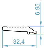
code :604 پروفیل تاسکوز آلومینیومی Glass Support Profile weight : 0.33 kg/m
