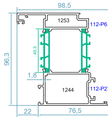
code : 1244-1253 لنگه درب داخل بازشو inward opening door weight 2.52 kg/m
