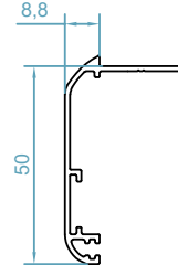
code :2500 پروفیل روکوب Border Profile weight : 0.38 kg/m
