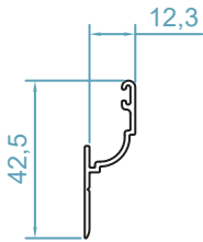
code :2508 ریل توری کشویی rail profile weight 0.23
