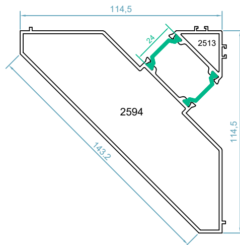
code : 2549 فریم توری پلیسه Fly Screen Frame weight : 0.43 kg/m
