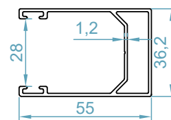
ریل آکا Aka Rail Profile code: 9155
