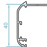
code : 2501 پروفیل روکوب Border Profile weight : 0.35kg/m
