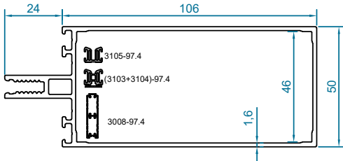
code : 3056 پروفیل افقی Transom Profile هم راستا با عمودی 3004 weight :1.87kg/m J_x=24.1 \text{ cm}^4 J_y=120.01 \text{ cm}^4
