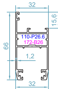
code : 2056 لنگه زهوار دار sash profile weight : 0.83 kg/m
