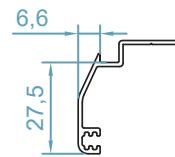
code :2524 پروفیل روکوب border profile weight 0.27 kg/m
