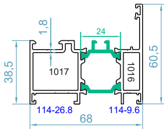
code : 1016-1017 پروفیل فریم frame profile weight 1.66 kg/m J_x=31 \text{ cm}^4 J_y=12 \text{ cm}^4
