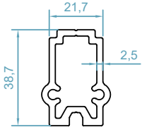
code :2289 ثابت کننده و آداپتورمونو ریل fixing profile weight :0.98 kg/m
