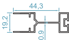
code : 2548 لنگه توری پلیسه fly screen sash weight :0.440 kg/m
