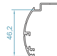
code :2522 پروفیل روکوب border profile weight 0.37 kg/m
