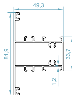
code : 1580 پروفیل سپری T Profile weight : 1.02 kg/m
