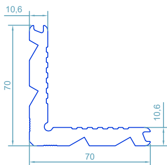
code : 110 گونیا پانچی corner cleat weight : 3.32kg/m
