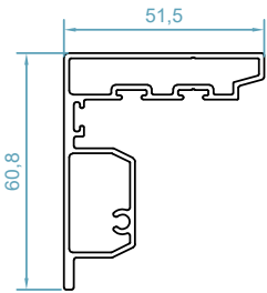
code :2297 آداپتور سه لنگه وسط باز شو fixing profile weight : 1 kg/m
