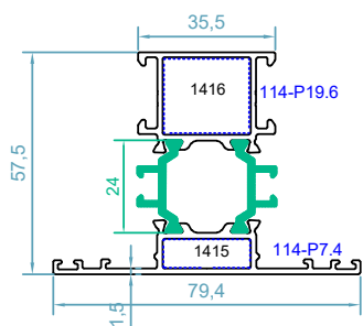
code : 1415-1416 سپری و بازشو محوری Pivoting Profil weight : 1.45 kg/m J_x = 18.8 \text{ cm}^4 J_y = 12.9 \text{ cm}^4
