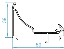
code : 2518 آداپتور گردان فریم 1501 Corner Adapter 1501 weight :0.57 kg/m
