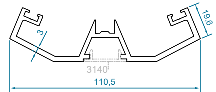
code : 3141 درپوش کنج بیرونی 135° Corner Cover Cap 135° weight : 1.76kg/m
