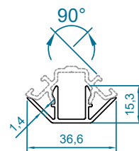
code : 3135 درپوش کنج داخلی 90° Corner Cover Profile 90° weight : 0.32kg/m
