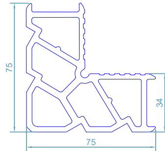
code : 121 گونبای پانچی Corner Cleat weight : 3.8kg/m
