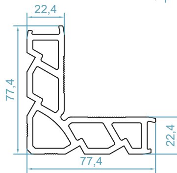
code : 114 گونیا پانچی corner cleat weight 3.67kg/m
