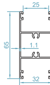
code : 2100 سپری لنگه بدون زهوار T profile for sash weight : 0.79 kg/m
