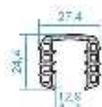
code :674 لاستیک تنظیم 13.5mm GLAZING ADJUSTING U GASKET 246 gram/metr
