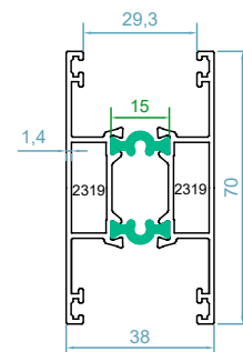
code : 2319-2319 سپری بدون زهوار T profile weight :1.12 kg/m J_x=14.5 \text{ cm}^4 J_y=9.12 \text{ cm}^4
