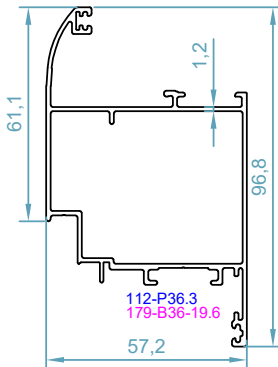
code : 1541 درب داخل بازشو Inward Opening Door Sash weight : 1.15 kg/m
