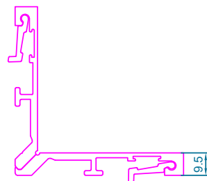
code:PC B9/5N گونیا آلنی لنگه طول برش 34.5 میلی متر
