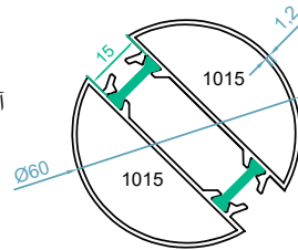
code : 1015-1015 1005-1006 آداپتور کنج فریم 1005-1006 Corner Adapter weight :1.78 kg/m J_x=12.02 \text{ cm}^4 J_y=12.11 \text{ cm}^4
