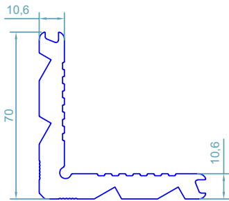
code : 110 گونیای پانچی Corner Cleat weight : 3.32kg/m
