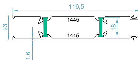
code : 1445-1445 ورق دو جداره ی ترمال بریک Thermal Break Fshutter Pro weight : 1.450 kg/m
