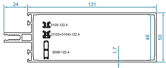
code : 3055 پروفیل افقی Transom Profile هم راستا با عمودی 3003 weight :2.19kg/m J_x=30.13 \text{ cm}^4 J_y=199.79 \text{ cm}^4
