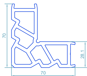
code : 102 گونیای پانچی Corner Cleat weight : 3.6kg/m
