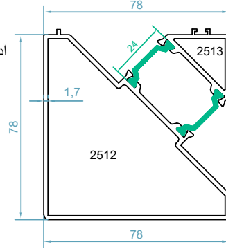
code :2512-2513 1006-1009 آداپتور کنج فریم 1006-1009 Corner Adapter weight : 2.1kg/m J_x=58.7 \text{ cm}^4 J_y=51.8 \text{ cm}^4
