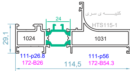
code :1024-1031 پروفیل فریم frame profile weight 1.90 kg/m
