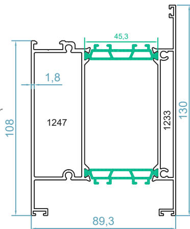
code : 1020-1256 اداپتور درب بیرون بازشو outward opening adapter weight 1.68 kg/m
