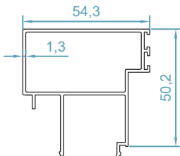
code : 2298 درپوش لنگه مخفی مونوریل frame cover weight : 0.811 kg/m
