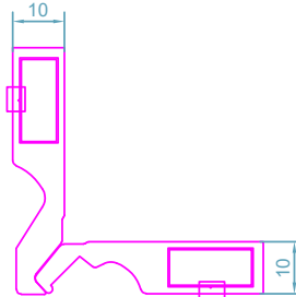
code : 176 PC B10 گونیای آلنی فریم و لنگه طول برش در اندازه های مختلف
