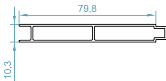
code : 2589 ورق تک جداره Shutter Profile weight : 0.64 kg/m
