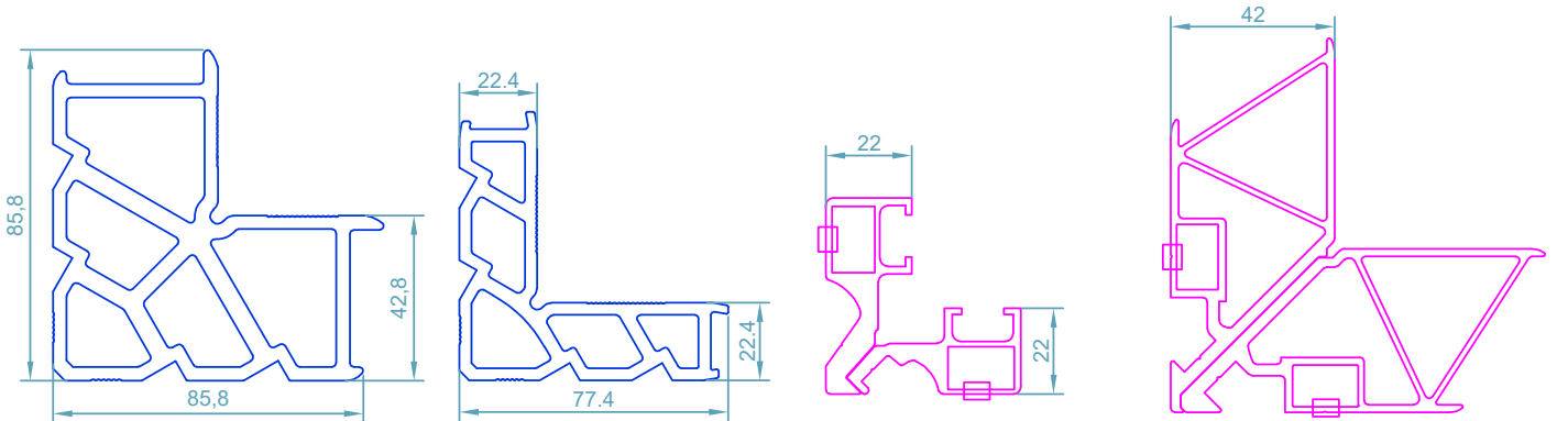
code : 112 گونیای پانچی Corner Cleat weight : 5.00 kg/m
