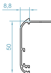
code : 2500 پروفیل روکوب Border Profile weight : 0.38kg/m
