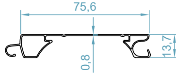
تیغه تک جداره رو به داخل Single Sheet Shutter code: 9001
