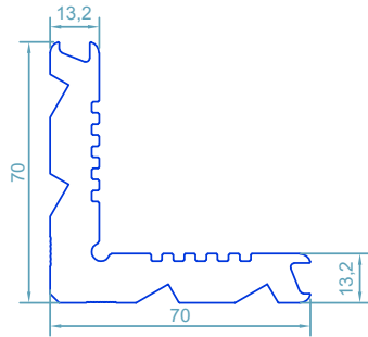
code : 111 گونیای پانچی Corner Cleat weight : 4.03kg/m
