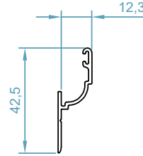
code : 2508 ریل توری کشویی Rail Profile weight : 0.23 kg/m
