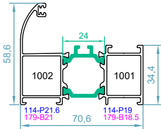
code : 1001-1002 پروفیل فریم Frame Profile weight : 1.32 kg/m
