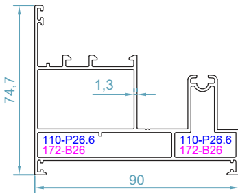
code : 2013 فریم مونوریل monorail frame weight : 1.716 kg/m
