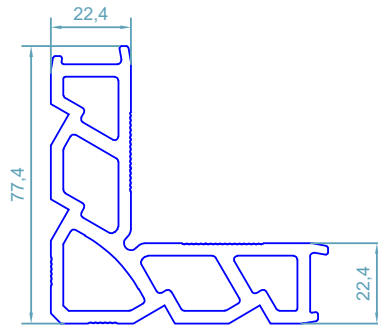
code : 114 گونیای پانچی Corner Cleat weight : 3.67 kg/m
