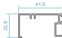
code : 2295 کاور فریم Cover Profile weight : 0.36 kg/m
