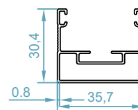
code : 2549 فریم توری پلایسه Fly Screen Frame weight : 0.43 kg/m
