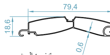
تیغه الون Eleven Shutter
