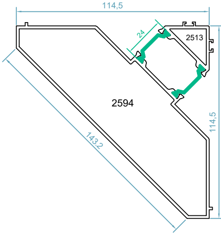
code :2513-2594 1006-1014 آداپتور کنج فریم 1006-1014 Corner Adapter weight :2.70 kg/m
