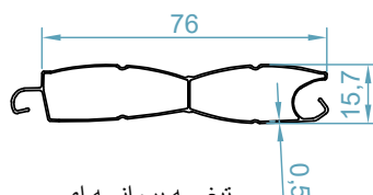
تیغه پروانه ای Butterfly New Shutter
