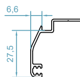
code : 2524 پروفیل روکوب Border Profile weight : 0.27 kg/m
