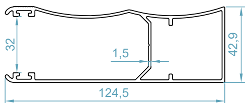
ریل نوبل Noble Rail Profile code: 9150
