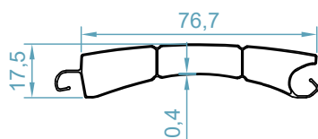
تیغه هلگورد Helgord Shutter
