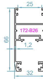
code : 2055 لنگه ی بدون زهوار sash profile weight : 0.92 kg/m
