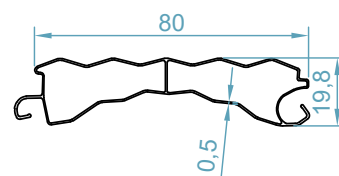
تیغه کرش Crash Shutter
