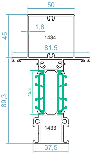
code : 1433-1434 سپری تقویت شده suprted mullion pr weight 2.96 kg/m
