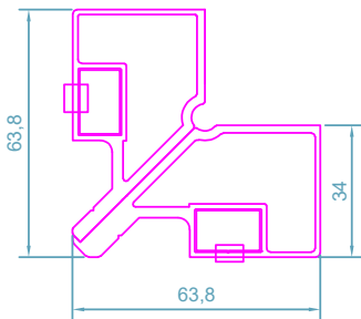
code : L34 (ALFIT) گونبای آلفی Corner Cleat قابل تولید در اندازه های مختلف
