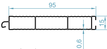
تیغه انتهایی End Shutter code: 9100
