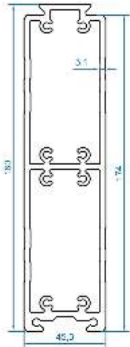
code : 3008 پروفیل انبساط عمودی Dilatation Profile weight : 4.960 kg/m
