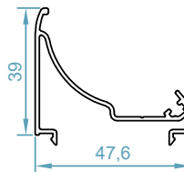
code : 1508 آداپتور گردان فریم 1500 Corner Adapter 1500 weight :0.48 kg/m
