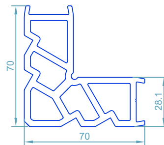
code : 102 گونیای پانچی Corner Cleat weight : 3.60 kg/m
