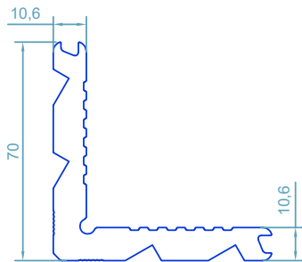
code : 110 گونیای پانچی Corner Cleat weight : 3.32kg/m
