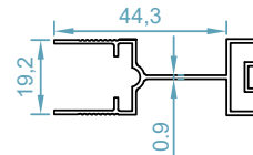
code : 2548 لنگه توری پلایسه Fly Screen Sash weight : 0.44 kg/m
