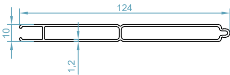
code : 2520 ورق تک جداره Shutter Profile weight : 0.82 kg/m
