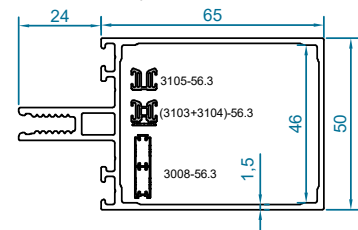
code : 3058 پروفیل افقی Transom Profile weight :1.53kg/m J_x=14.4 \text{ cm}^4 J_y=42.4 \text{ cm}^4
