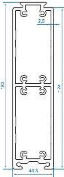
code : 3012 3013,3010 پروفیل انبساط برای عمودی Dilatation Profile weight : 4.800 kg/m
