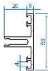
code : 3102 Add On پروفیل Add On Profile weight : 0.700 kg/m
