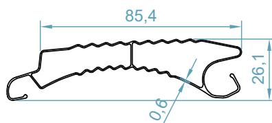
تیغه پاکر Pucker Shutter
