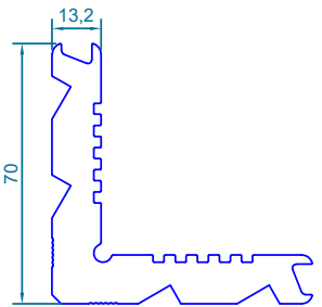
code : 111 گونیا پانچی لنگه ی بدون زهوار Corner Cleat weight : 4.03 kg/m
