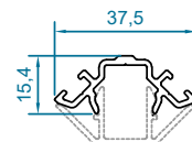
code : 3134 نگهدارنده ی کنج داخلی 90° Corner Presuure Plate 90° weight : 0.34kg/m
