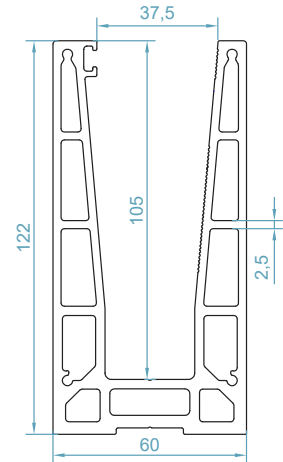
سیستم نرده شیشه ای HUCK 122
