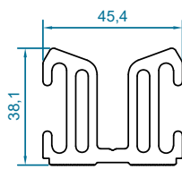
code : 3105 كانكتور فيكس Transom Joint Profile weight :2.14kg/m
