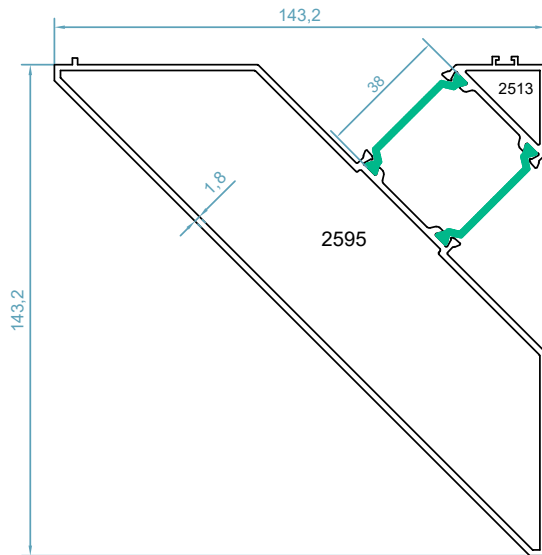
code : 2513-2595 آداپتور کنج فیکس مونوریل corner adaptor weight : 3.18kg/m
