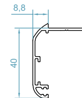
code : 2501 پروفیل روکوب Border Profile weight : 0.35kg/m
