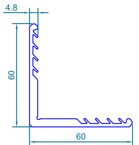
code : 119 گونیا آلومینیومی فشاری فریم کوتاه Aluminium Force Fitting Corner weight : 1.20 kg/m ALUMINIUM
