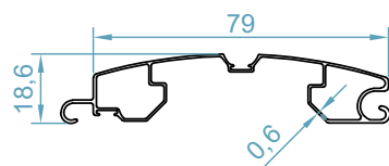
تیغه الون پنچ Eleven Punch Shutter
