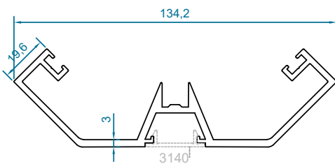
code : 3142 درپوش کنج بیرونی 90° Corner Cover Cap 90° weight : 2.0kg/m
