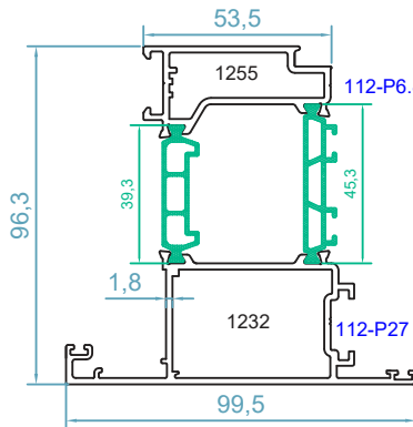
code : 1232-1255 لنگه درب بیرون بازشو outward opening door weight 2.51 kg/m
