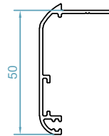
code : 2500 پروفیل روکوب Border Profile weight : 0.38kg/m
