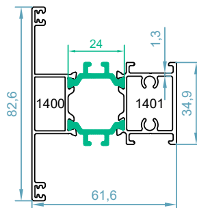
code : 1400-1401 پروفیل سپری T Profile weight : 1.42 kg/m
