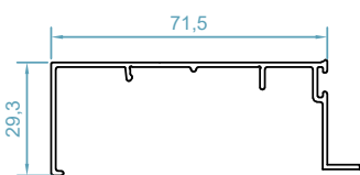
code : 2286 کاور فریم بلند cover profile weight :0.550 kg/m
