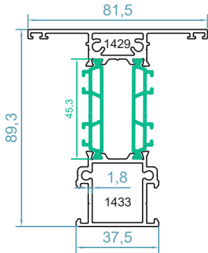
code : 1429-1433 سپری فریم و لنگه transom-mullion profile weight 2.12 kg/m
