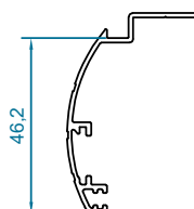
code :2522 پروفیل روکوب Border Profile weight : 0.37 kg/m
