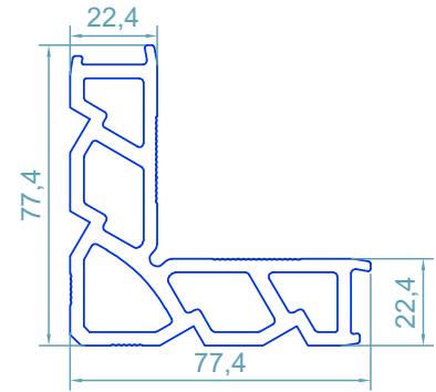
code : 114 گونیا پانچی Corner Cleat weight : 3.67kg/m
