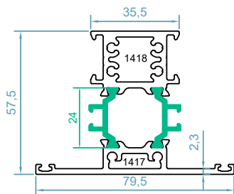
code : 1417-1418 سپری تقویت شده Supported T Profile weight : 2.15 kg/m J_x = 27.04 \text{ cm}^4 J_y = 17.02 \text{ cm}^4
