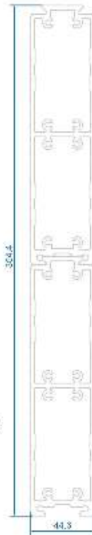
code : 3012 3013,3010 پروفیل انبساط برای عمودی Dilatation Profile weight : 4.800 kg/m
