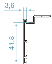
code :2523 پروفیل روکوب border profile weight 0.32 kg/m
