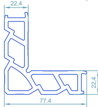
code : 114 گونیای پانچی Corner Cleat weight : 3.67 kg/m
