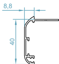
code :2501 پروفیل روکوب Border Profile weight : 0.35 kg/m
