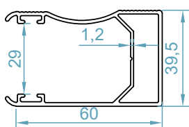
ریل سانی Sunny Rail Profile code: 9153
