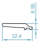
code : 604 پروفیل تاقوز آلومینیومی Galss Support Profile weight : 0.35 kg/m
