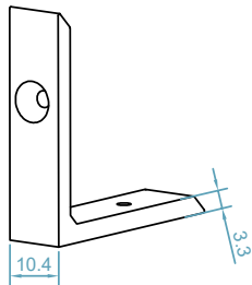
code : 120 گونیای آلومینیومی فریم های کوتاه Low Frame Corner Cleat
