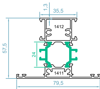
code : 1411-1412 پروفیل سپری T Profile weight : 1.5 kg/m J_x = 20.6 \text{ cm}^4 J_y = 13.02 \text{ cm}^4
