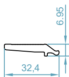
code : 604 پروفیل تاقوز آلومینیومی Glass Support Profile weight : 0.35 kg/m
