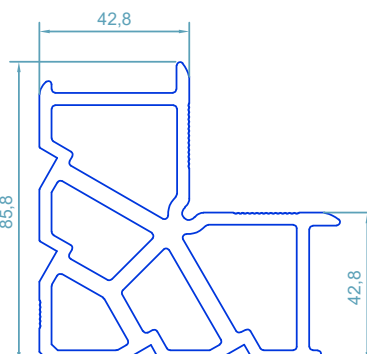
code : 112 گونیای پانچی Corner Cleat weight : 5kg/m
