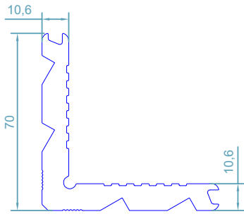
code : 110 گونیبا پانچی Corner Cleat weight : 3.32 kg/m
