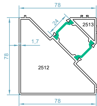
code : 2512-2513 آداپتور کنج فریم Corner Adapter weight : 2.1kg/m
