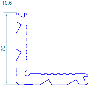
code : 110 گونیا پانچی فریم Corner Cleat weight : 3.32 kg/m
