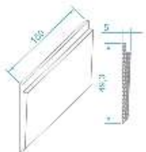
code : 629 پلاستیک نصب شیشه 19.5mm GLAZING WEDGE
