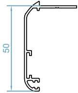
code :2500 پروفیل روکوب Border Profile weight : 0.38kg/m
