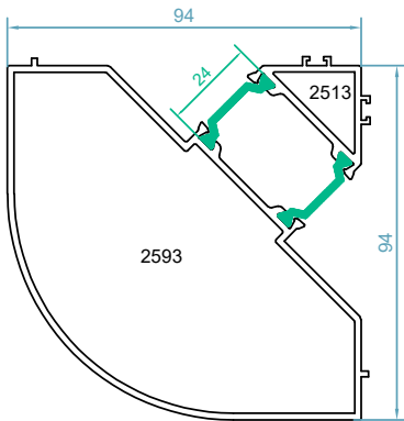
code :2513-2593 1006-1026 آداپتور کنج فریم 1006-1026 Corner Adapter weight :2.40 kg/m
