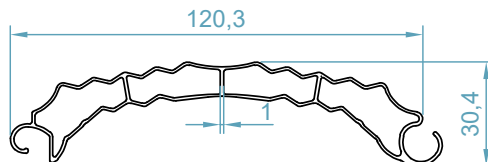
تیغه ارنست Ernest Shutter
