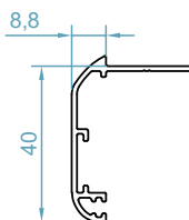
code : 2501 پروفیل روکوب Border Profile weight : 0.35kg/m
