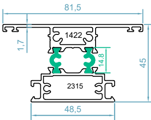
code : 1422-2315 سپری دو طرف شیشه T profile weight :1.72 kg/m Jx=18 \text{ cm}^4 Jy=15 \text{ cm}^4
