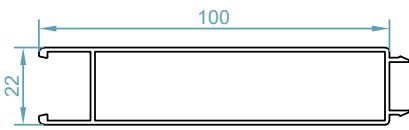
code : 2511 ورق دو جداره Shutter Profile weight : 1.07 kg/m
