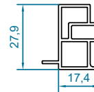
code : 2607 آداپتور ورق کامپوزیت Composite Panel Adapter weight :0.45kg/m
