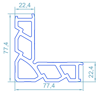
code : 114 گونیا پانچی Corner Cleat weight : 3.67kg/m
