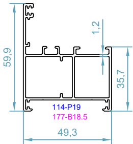
code : 1500 پروفیل فریم Frame Profile weight : 0.91 kg/m
