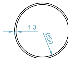
code : 2526 لوله گردان فریم 1500 Corner Adapter 1500 weight :0.55 kg/m
