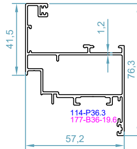
code : 1542 پنجره داخل بازشو Inward Opening Window weight : 1.05 kg/m
