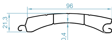
تیغه قوس 100 Curve 100 Shutter
