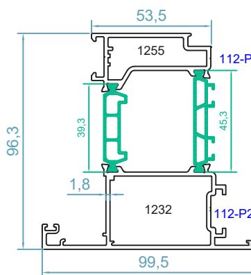
code : 1232-1255 لنگه درب بیرون بازشو outward opening door weight 2.51 kg/m
