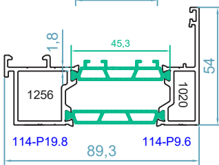
code : 1020-1256 اداپتور درب بیرون بازشو outward opening adapter weight 1.68 kg/m
