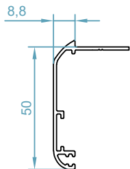
code :2500 پروفیل روکوب Border Profile weight : 0.38 kg/m
