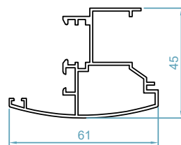
code : 1591 پروفیل اورهانگ Double Sash Adaptor weight : 0.76 kg/m Jx=5.46 \text{ cm}^4 Jy=5.69 \text{ cm}^4
