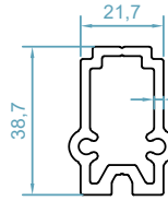
code :2289 کانتور نصب اسپر لنگه مونوریل 2262-2263 T Joint weight :0.98 kg/m
