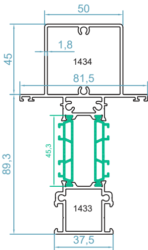
code : 1433-1434 سپری تقویت شده supported mullion pr weight 2.96 kg/m
