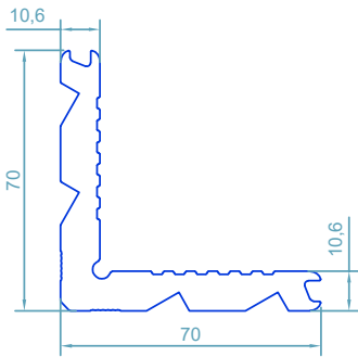
code : 110 گونیای پانچی Corner Cleat weight : 3.32kg/m
