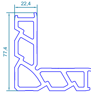
code : 114 گونیا پانچی Corner Cleat weight : 3.67kg/m
