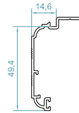
code : 2565 روکوب شیاردار Border Profile weight : 0.42kg/m
