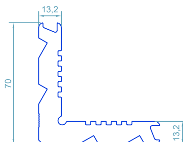
code : 178 PC B13 قابل تولید در اندازه های مختلف
