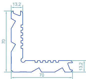
code : 111 گونیا پانچی corner cleat weight : 4.03kg/m
