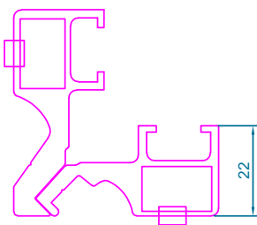
code : 119 گونیا آلومینیومی فشاری فریم کوتاه Aluminium Force Fitting Corner weight : 1.20 kg/m ALUMINIUM
