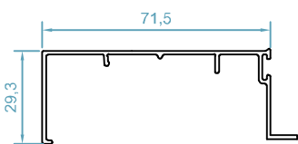
code : 2286 کاور فریم بانند cover profile weight : 0.550 kg/m
