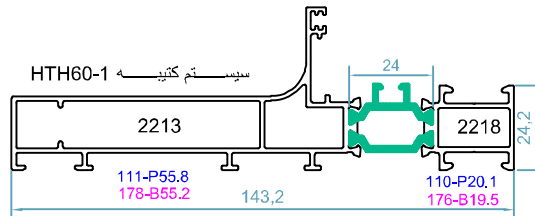
code : 2213-2218 کتیبه ی دوریل frame profile weight : 1.91 kg/m J_x = 136.5 \text{ cm}^4 J_y = 7.91 \text{ cm}^4
