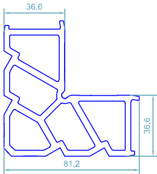
code : 106 گونیایا پانچی Corner Cleat weight : 4.250 kg/m
