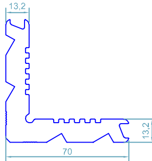
code : 111 گونیایا پانچی Corner Cleat weight : 4.03kg/m
