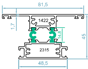
code : 1422-2315 سپری دو طرف شیشه T profile weight :1.72 kg/m Jx=18 cm 4 Jy=15 cm 4
