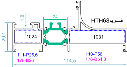
code :1024-1031 فریم کتیبه سری TH68 hinge adjoining frame weight : 1.90 kg/m
