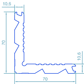
code : 110 گونیبا پانچی corner cleat weight : 3.32kg/m
