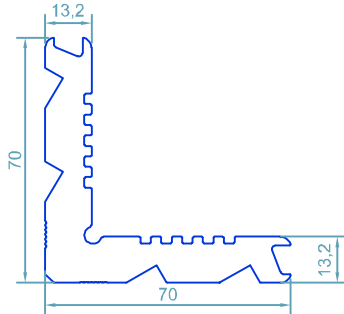
code : 111 گونیبا پانچی corner cleat weight : 4.03kg/m
