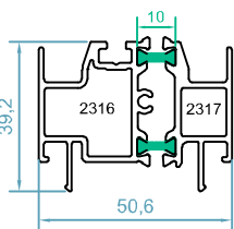
code : 2316-2317 آداپتور وسط چهار لنگه sash inversion profile weight :1.25 kg/m Jx=10.1 cm 4 Jy=5 cm 4
