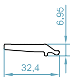
code : 604 پروفیل تاسکوز آلومینیومی Glass Support Profile weight : 0.35 kg/m
