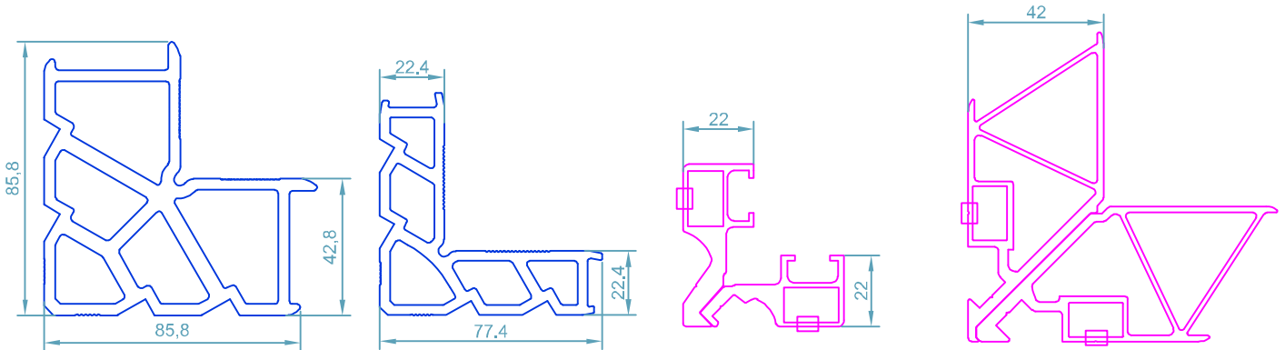
code : 112 گونیبا پانچی Corner Cleat weight :5.00 kg/m
