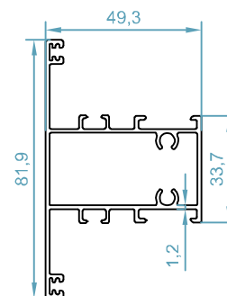
code : 1580 پروفیل T سبری T Profile weight : 1.02 kg/m
