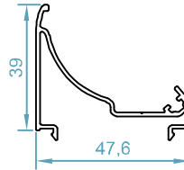
code : 1508 آداپتور گردان فریم 1500 Corner Adapter 1500 weight :0.48 kg/m
