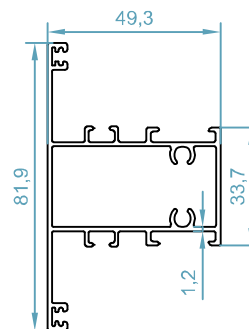
code : 1580 پروفیل T پری T Profile weight : 1.02 kg/m
