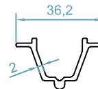
code : 2585 پروفیل ثابت کننده fixing profile weight : 0.36kg/m
