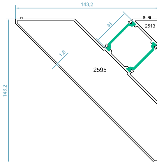
code : 2513-2595 آداپتور کنج فیکس مونوریل corner adaptor weight : 3.18kg/m
