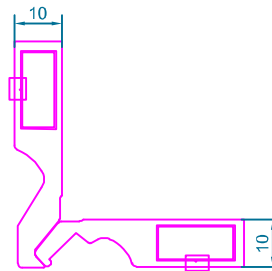
code : 176 PC B10 گونیا آلی فریم طول برش 26 میلی متر
