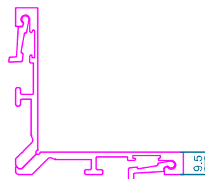
code:PC B9/5N گونیا آلی لنگه طول برش 34.5 میلی متر
