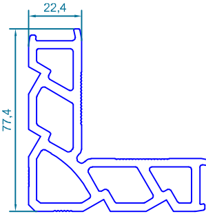
code : 114 گونیا پانچی Corner Cleat weight : 3.67kg/m
