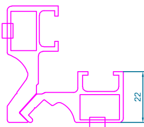
code : 119 گونیا آلومینیومی فشاری فریم کوتاه Aluminium Force Fitting Corner weight : 1.20 kg/m ALUMINIUM
